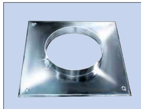
Piastra terminale di tenuta per rigido / flex con sistema di bloccaggio a bulloni.
